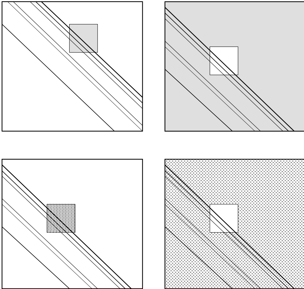
Ábra 2-1 A Henon-attraktor részlete (Az illusztráció az ismétlődő mintát mutatja.)
